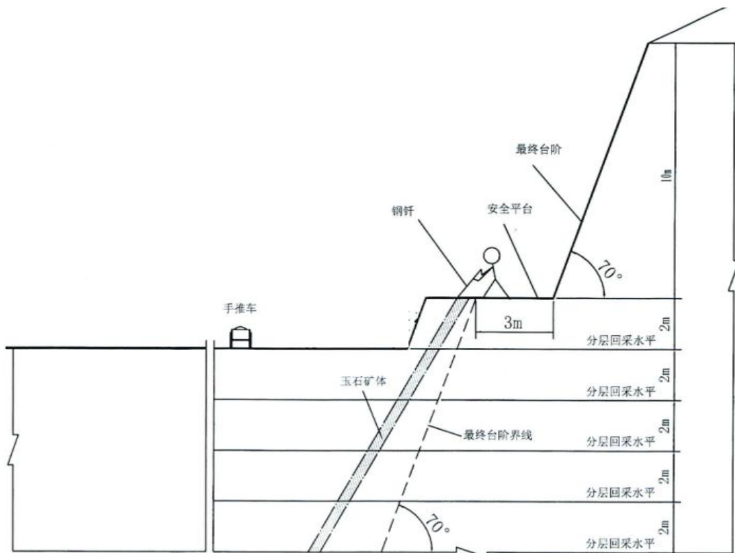
图 3.2-1 开采方法示意图
