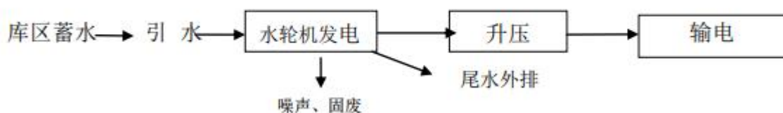
图4-1 水电站工艺流程及产污节点图
